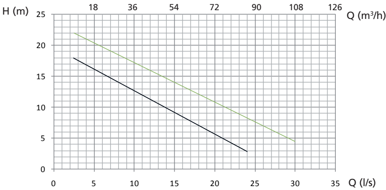
单泵运行曲线
