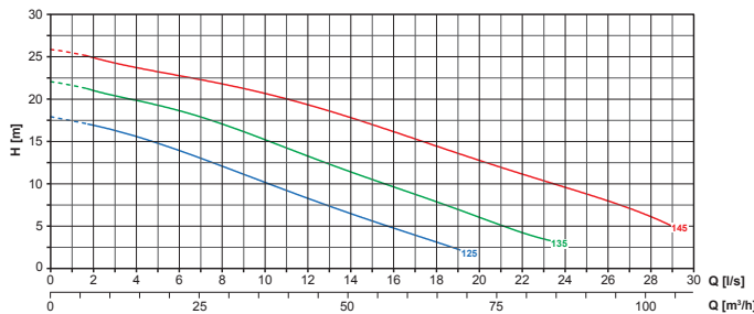
单泵运行曲线 BlueBox E 400S/ZUG V 065 A 5.5/2 A W BlueBox E 400S/ZUG V 065 A 7.5/2 A W BlueBox E 400S/ZUG V 065 A 9/2 A W
