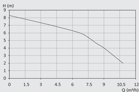
性能曲线
